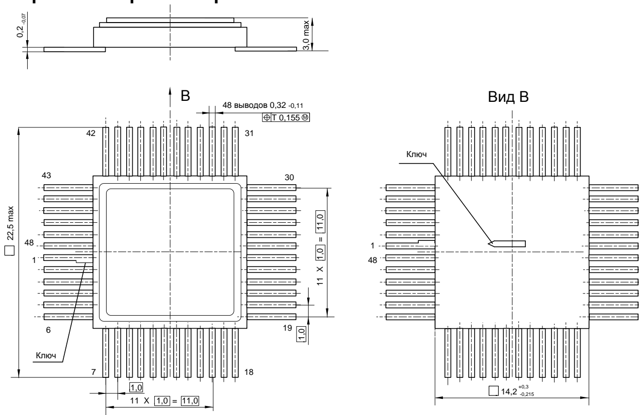
Рис.28 Габаритный чертёж микросхемы в корпусе N16.48-1B
