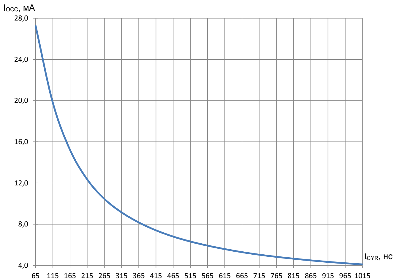
Рисунок 43 – Зависимость динамического тока потребления от времени цикла считывания информации t_{сцр} при U_{сс} = 3,6 В и T = 25 °С
