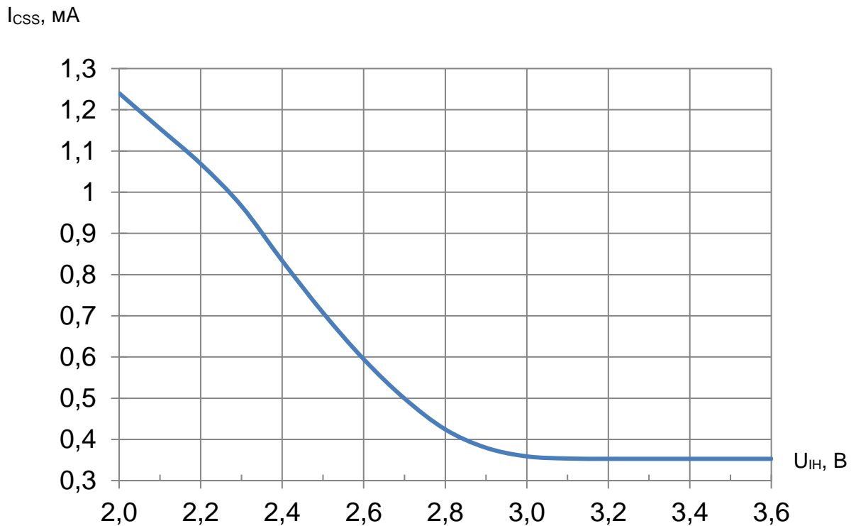
Рисунок 38 – Зависимость тока потребления в режиме хранения от входного напряжения высокого уровня при U_{CC} = 3,6\text{ V} , U_{IL} = 0\text{ V} , f = 0\text{ МГц} , T = 25\text{ }^{\circ}\text{C}
