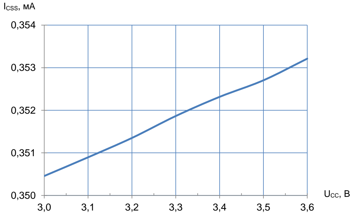
Рисунок 37 – Зависимость тока потребления в режиме хранения от напряжения питания при T = 25\text{ }^{\circ}\text{C}
