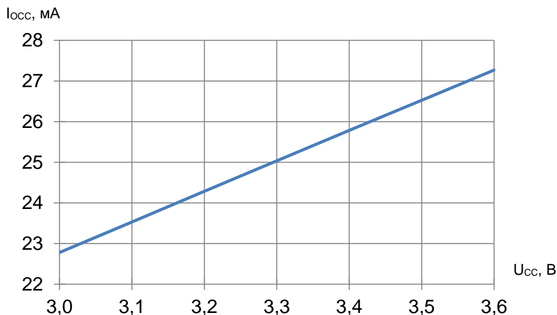
Рисунок 44 – Зависимость динамического тока потребления от напряжения питания при t_{сцр} = 70 нс, T = 25 °С
