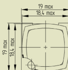
ПКБ502, ПКБ503, ПКБ504 (размеры - см. ПКБ501, ПКБ506)
